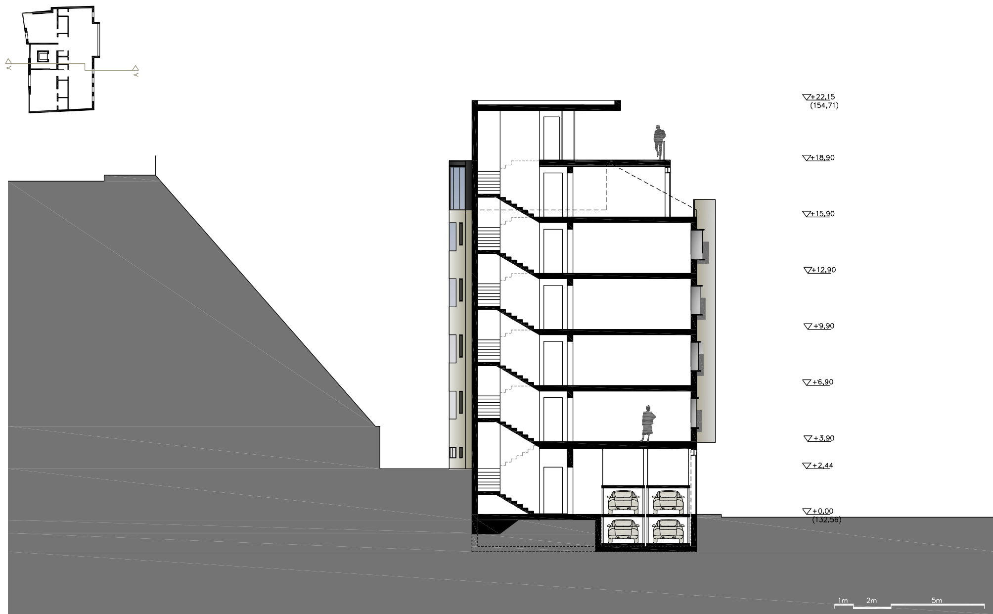
PRESJEK AA
