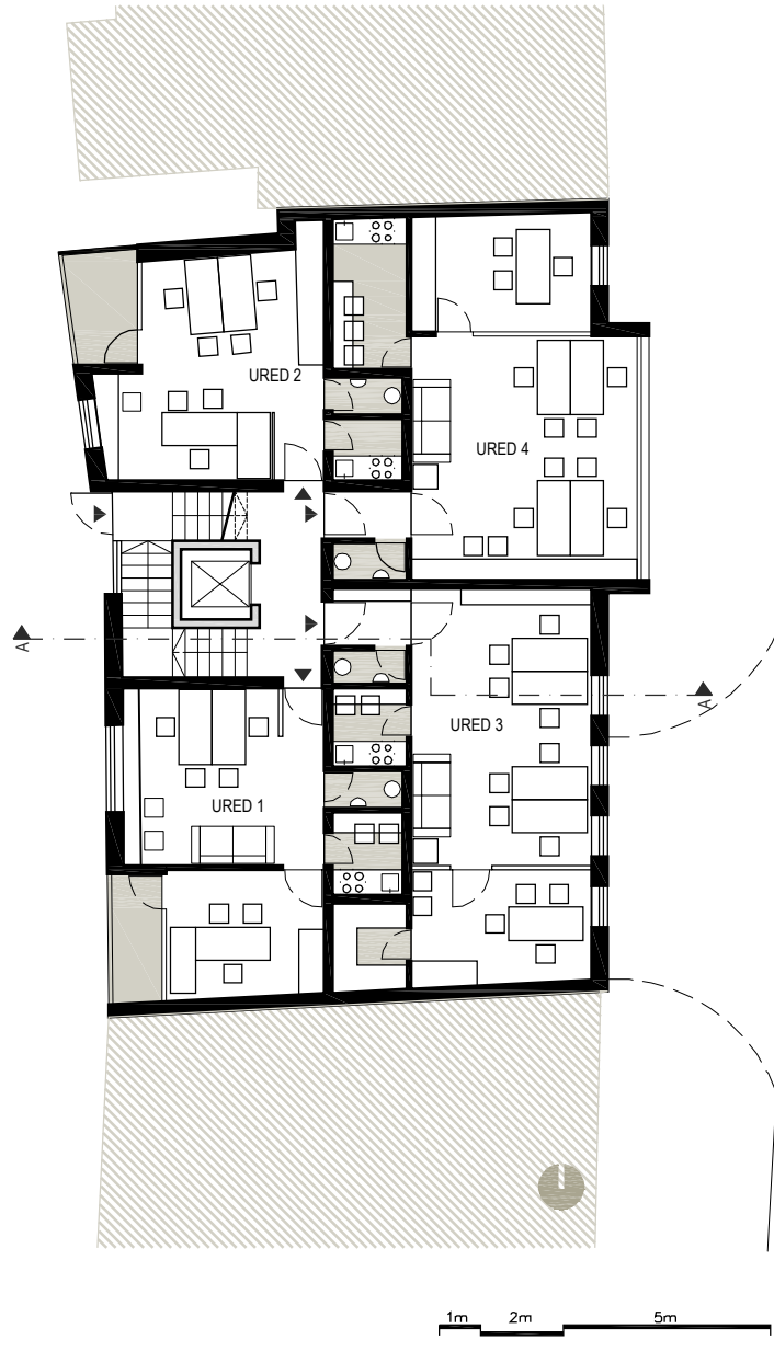
1. KAT (var. B - uredi) 1:200 P+1
