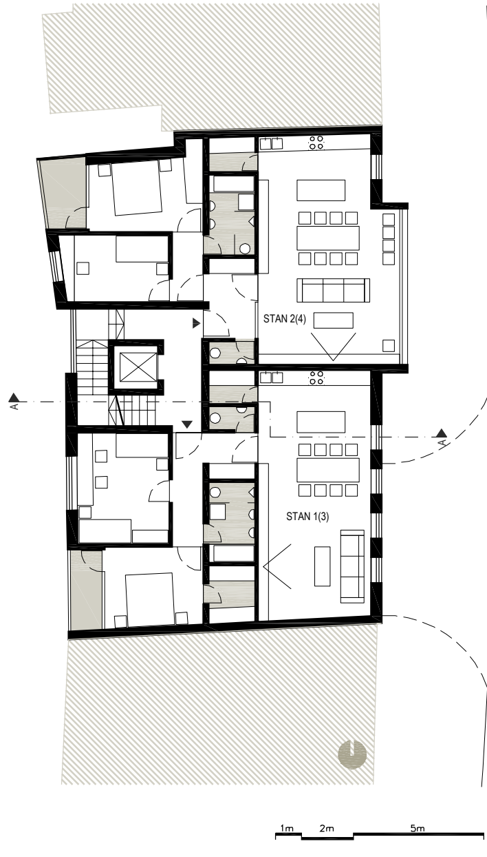
2,3,4. KAT (var. A) 1:200 P+2,3,4
