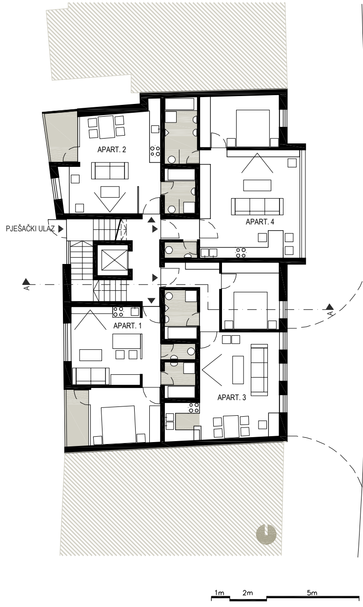
1. KAT (var. A - apartmani) 1:200 P+1
