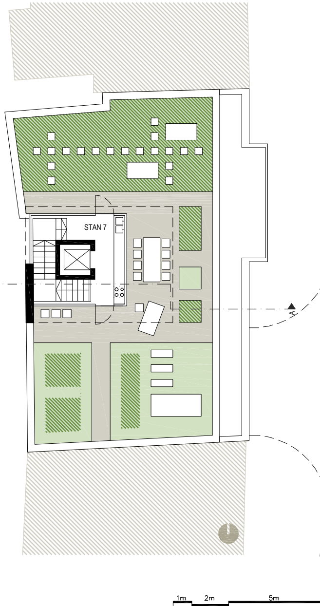
6. KAT, TERASA 1:200 P+6
