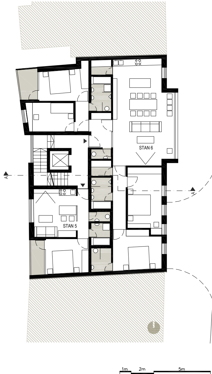
2,3,4. KAT (var. B) 1:200 P+2,3,4
