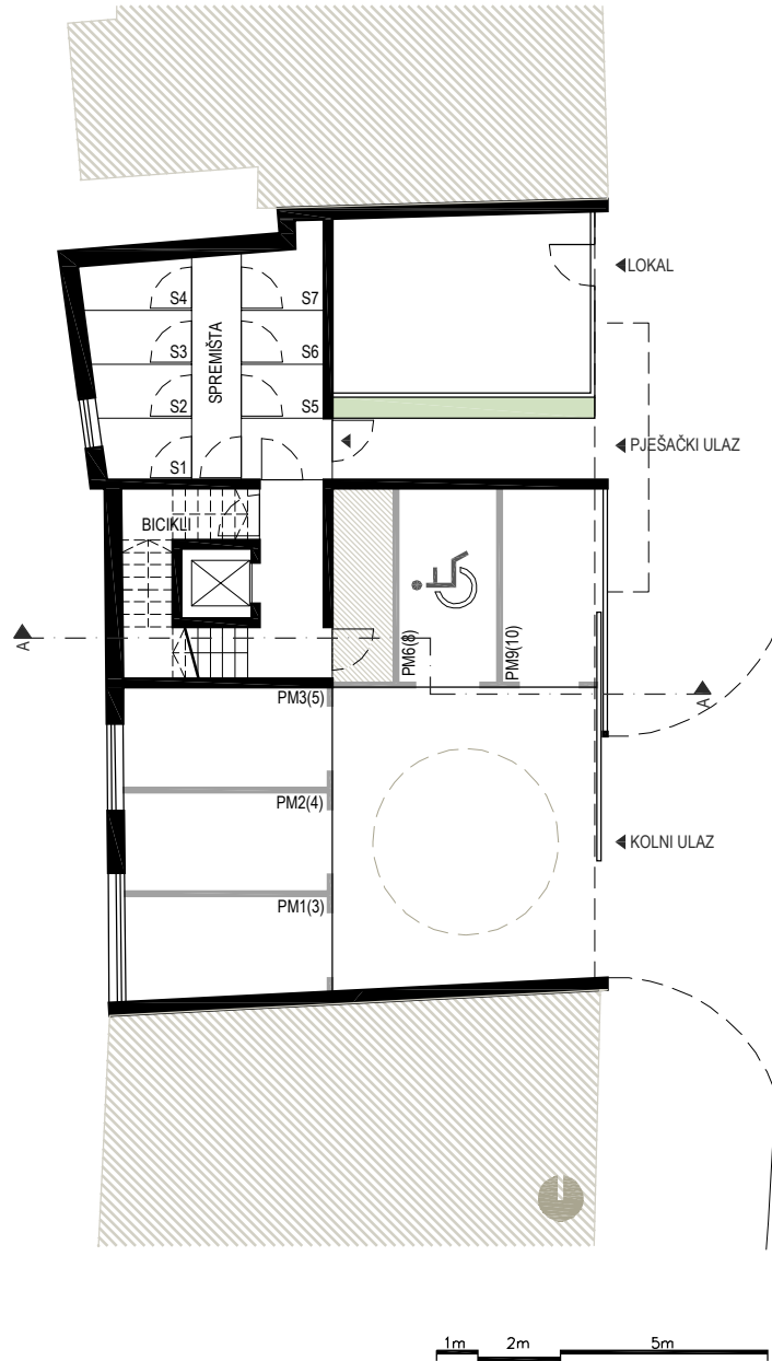
PRIZEMLJE 1:200 P
